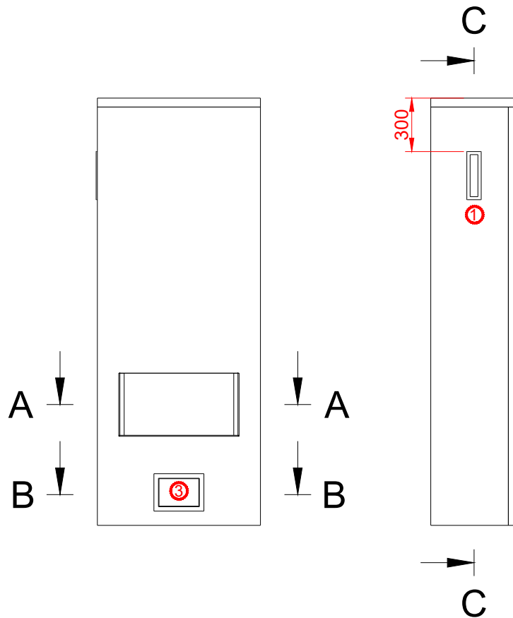
A-A (1:30)
