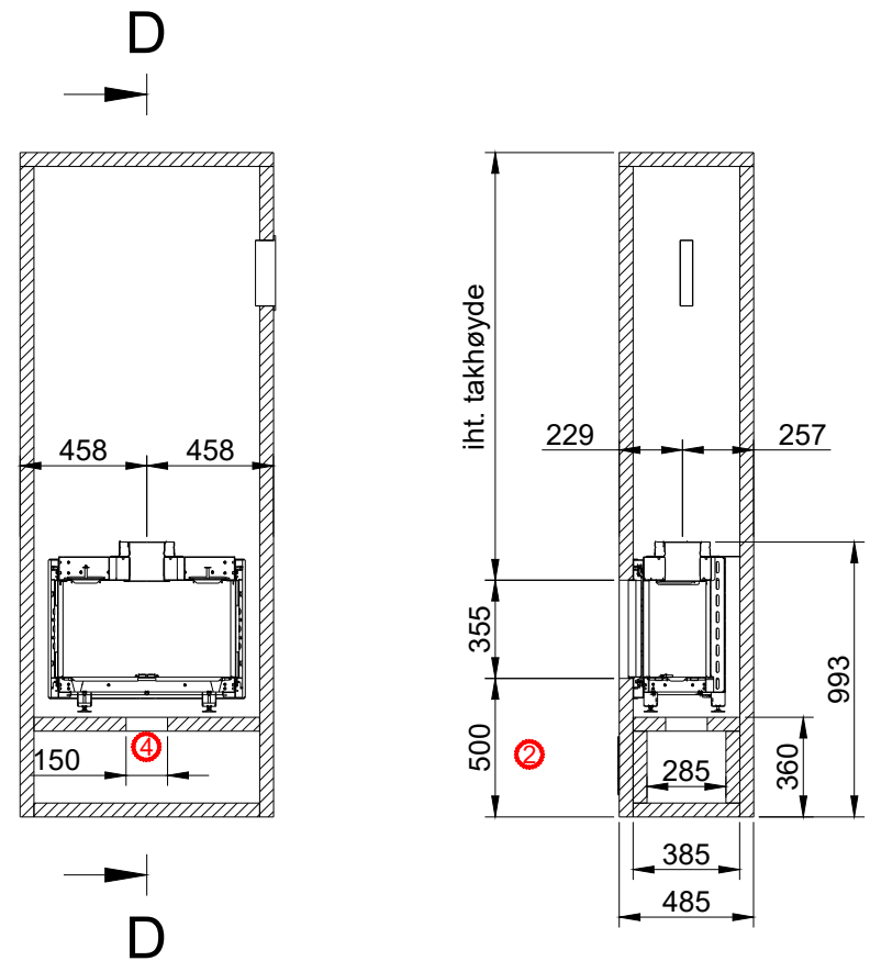
D-D (1:30)
