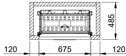
B-B (1:30)
